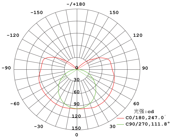
配光曲线
